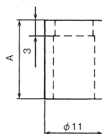
4mmねじ用カラー Collar for 4mm screw
