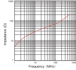
GTR-40-27-15
