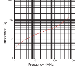
GTR-25-15-8
