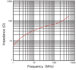
GTR-28-16-13
