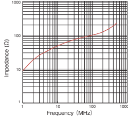
GTR-28-16-20
